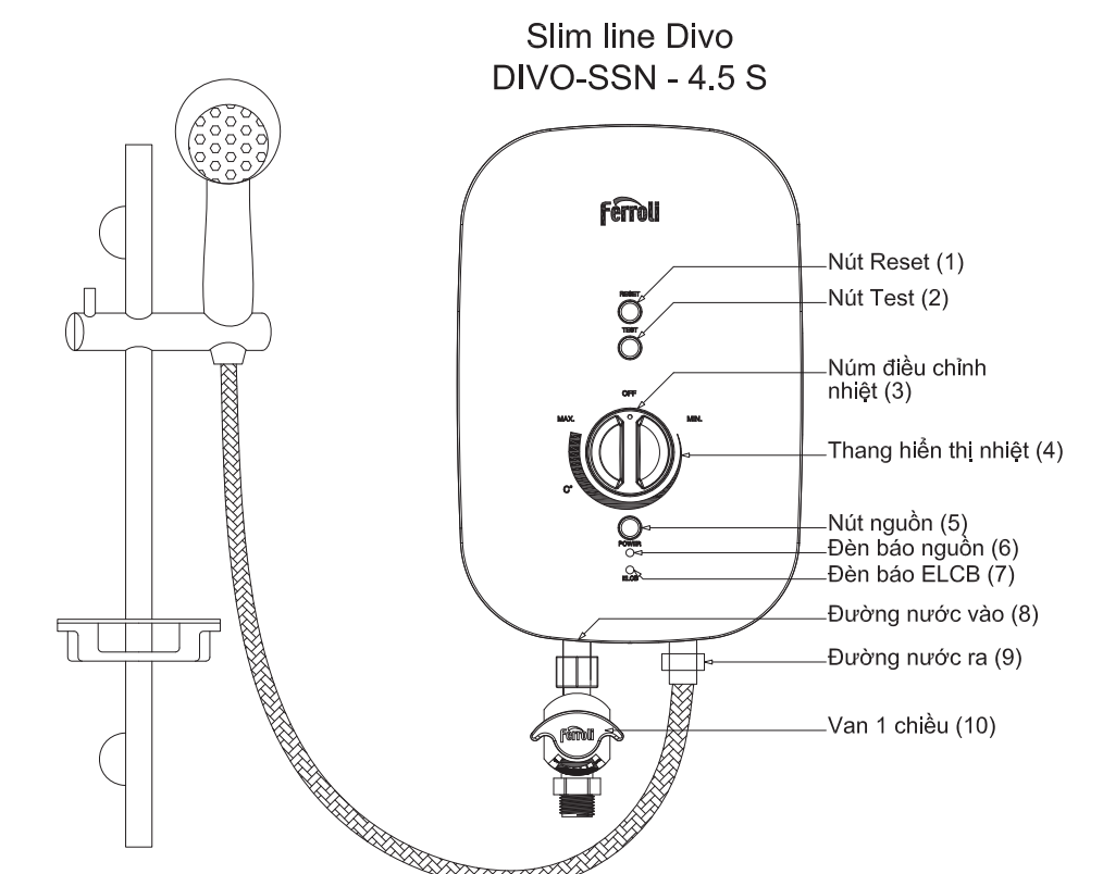
Hình 1. Mô tả máy nước nóng Slim line Divo SSN-4.5S
