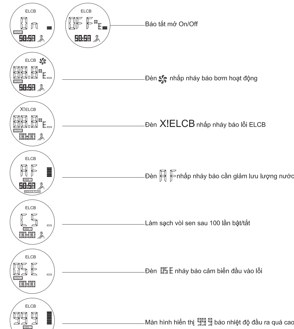
Hình 8. Các thông báo hiển thị của máy
