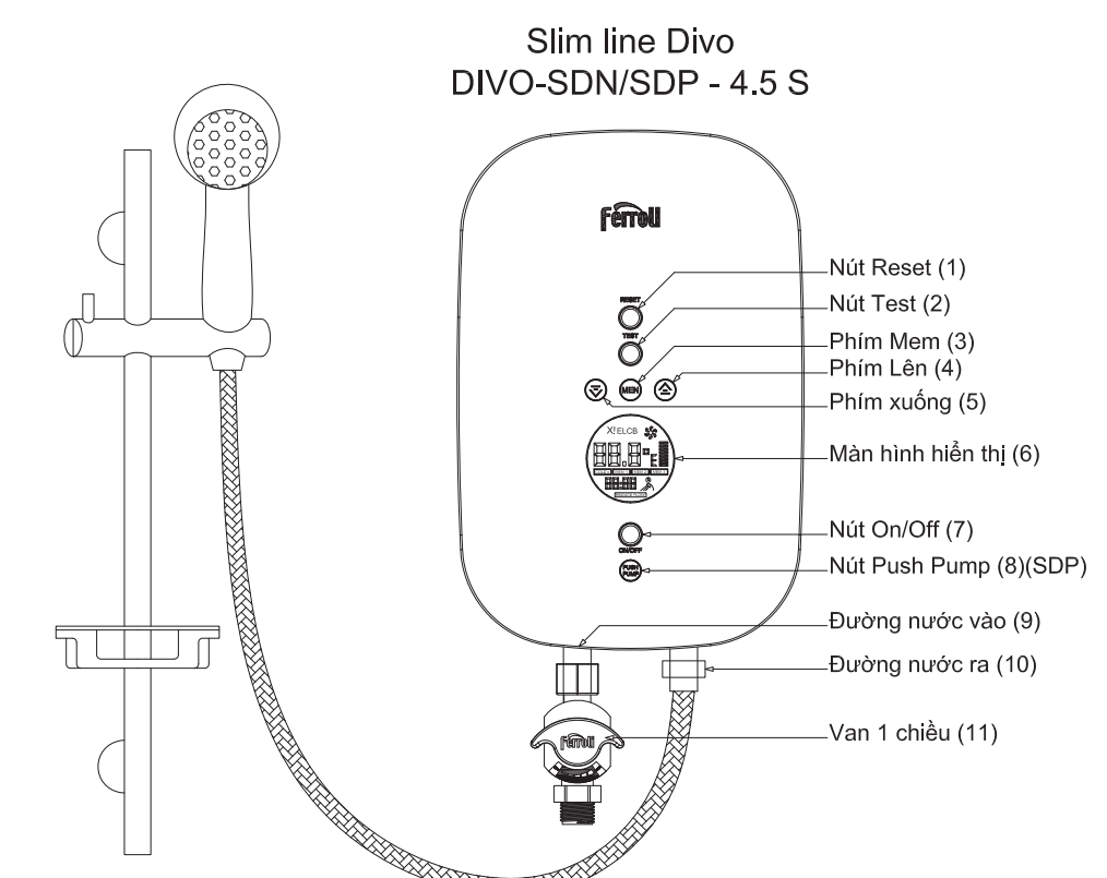
Hình 3. Mô tả máy nước nóng Slim line Divo SDN/SDP-4.5S
