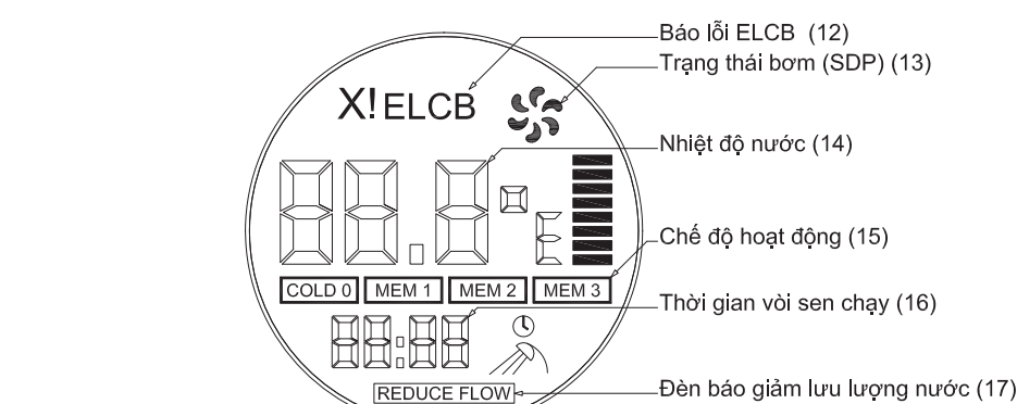
Hình 4. Màn hình hiển thị máy nước nóng SDN/SDP-4.5S
